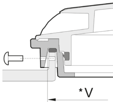
Seitenbefestigung
