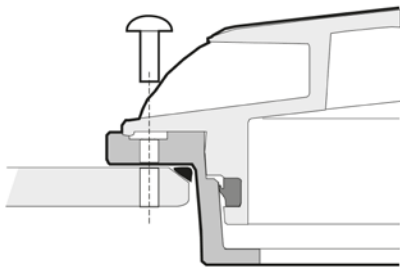
Obere Befestigung
